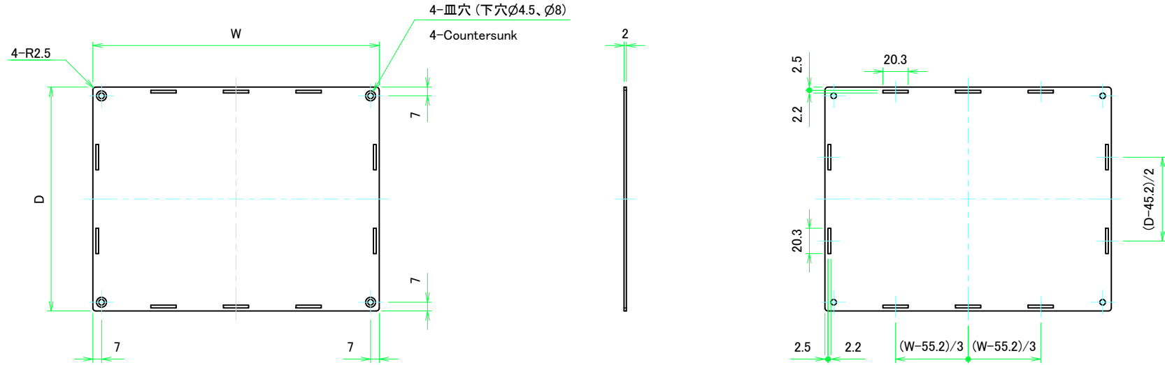
上カバー裏面 / Top cover Backside
