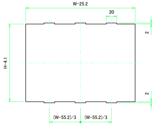
Wパネル1表面 / W Panel 1 Frontside
